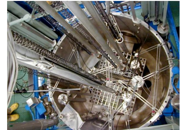
KUCAの炉心
